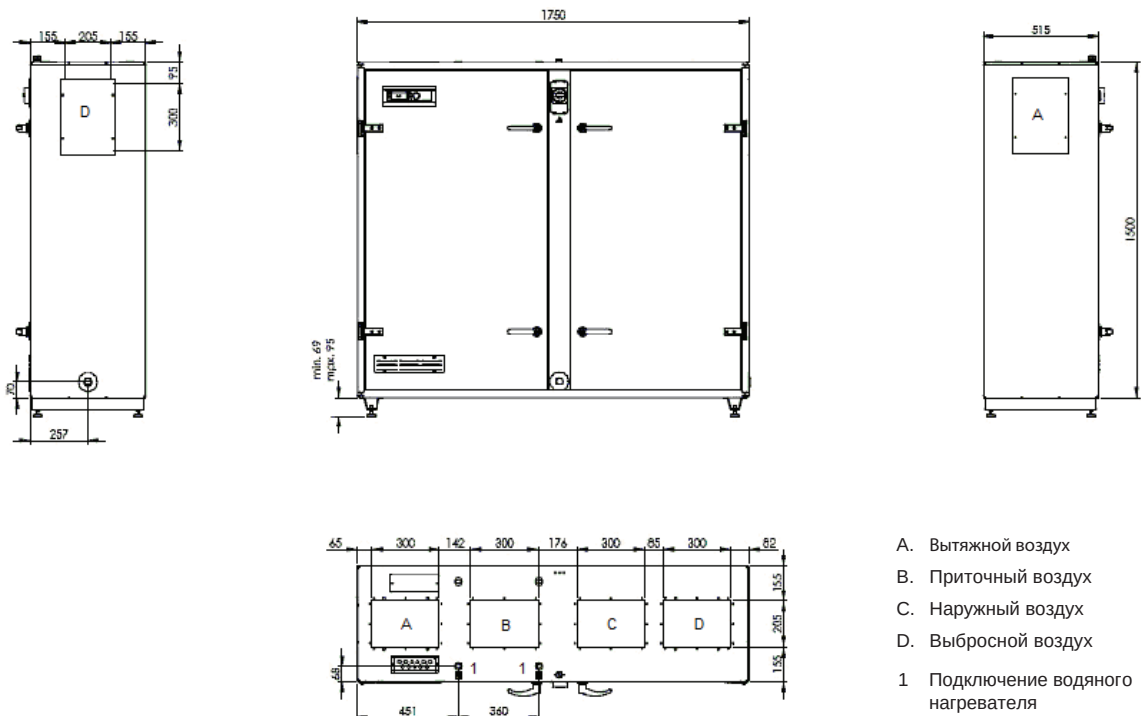
Установка показана в левостороннем исполнении
