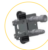
Устройство для подсоединения гибких шлангов от внешнего топливного бака BV 110, BV 170, BV 290 - 4034.880
